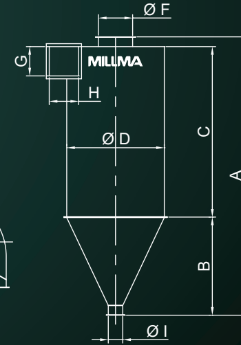
SAĞ / RIGHT
